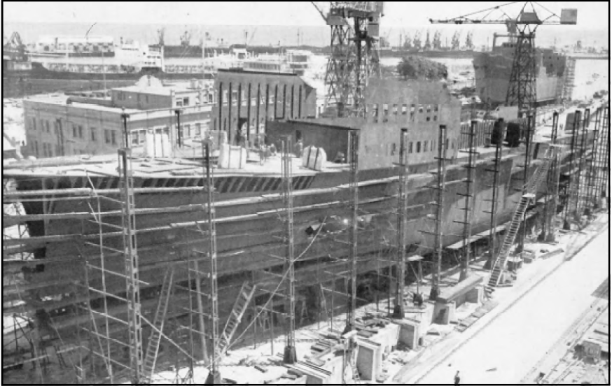
«Ciudad de Tarifa», el nuevo transbordador que se construye en la Unión Naval de Levante.
