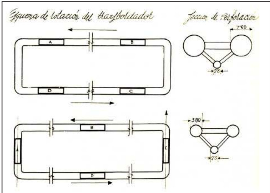
Esquema de rotación del transbordador propuesto por Goicoechea para el túnel del estrecho de Gibraltar.
